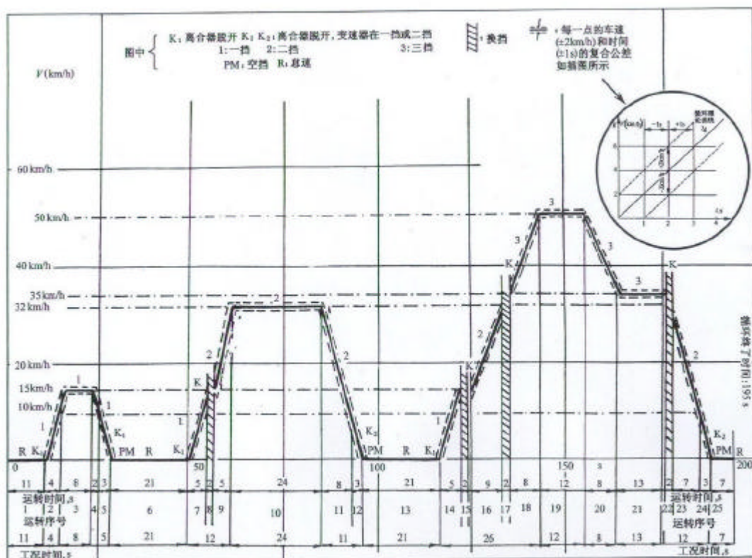
图 C.1 瞬态工况运转循环图
