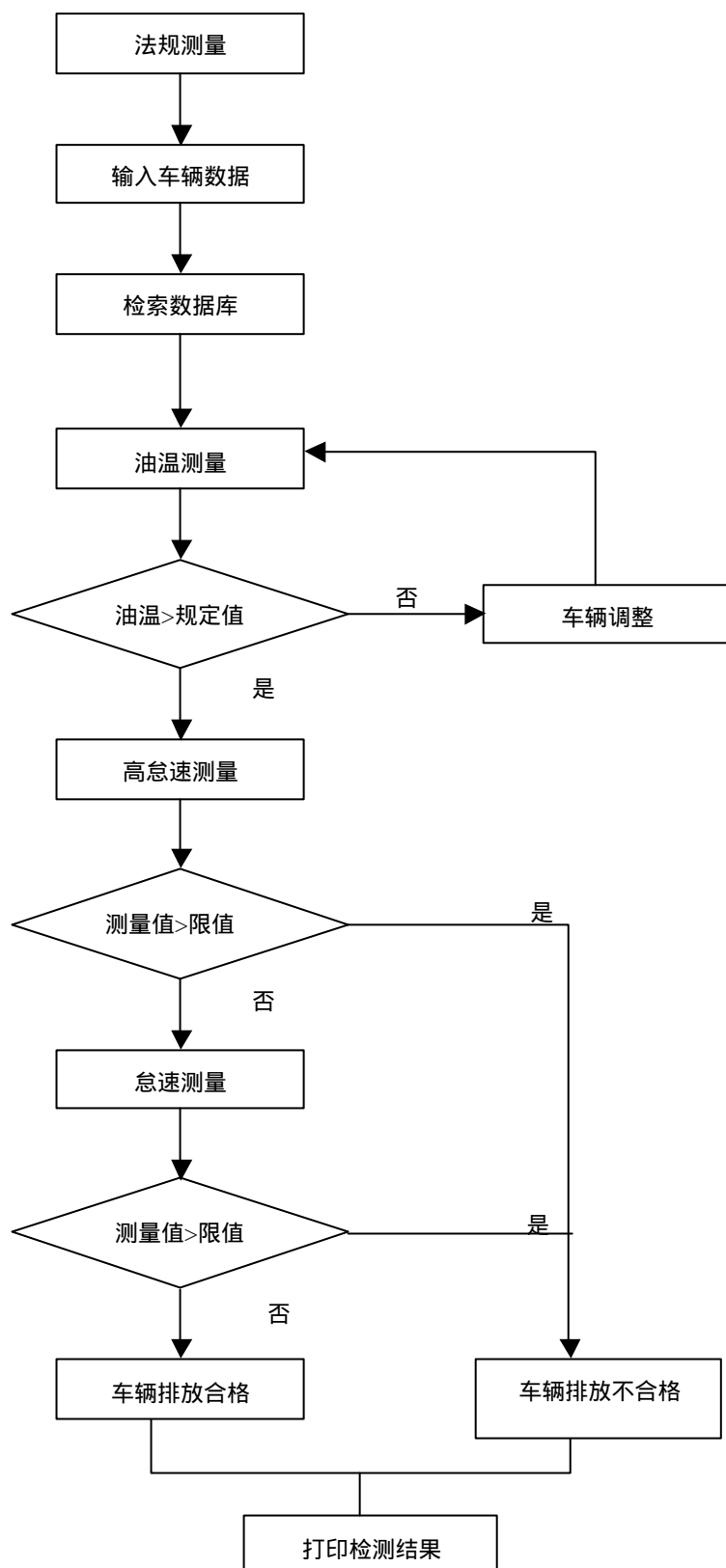
图 A.1 双怠速法仪器测量程序
