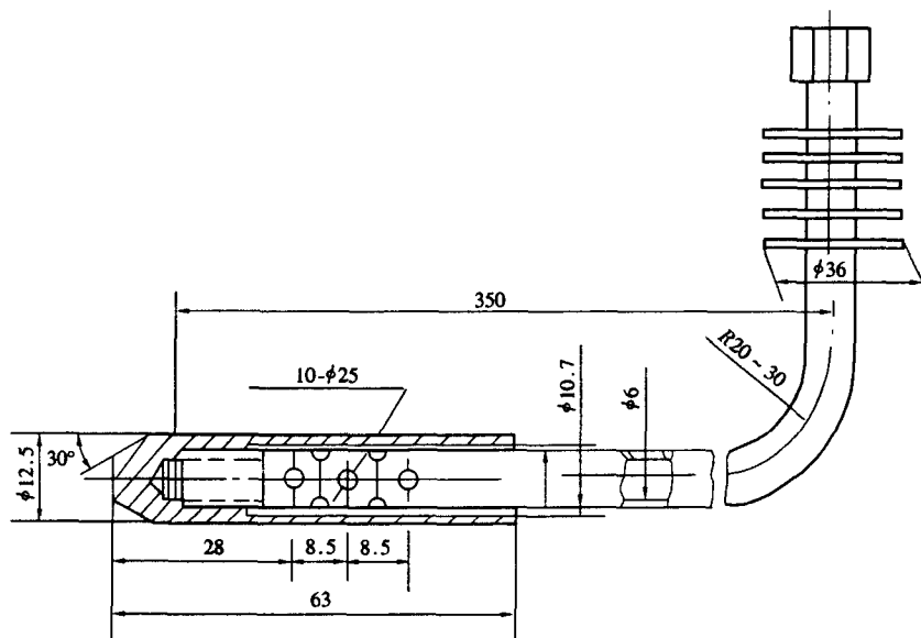
图 1 取样探头
